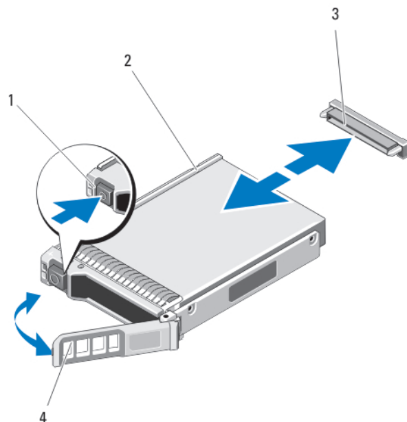
图 15: 卸下和安装硬盘驱动器/SSD
