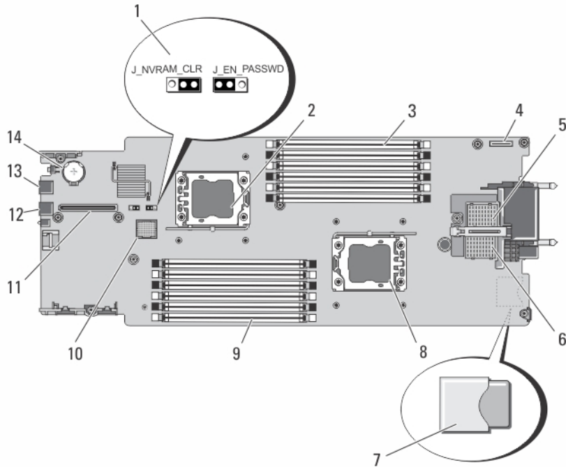
图 21: 系统板连接器
