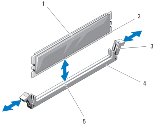
图 8: 安装和卸下内存模块或内存模块挡板
