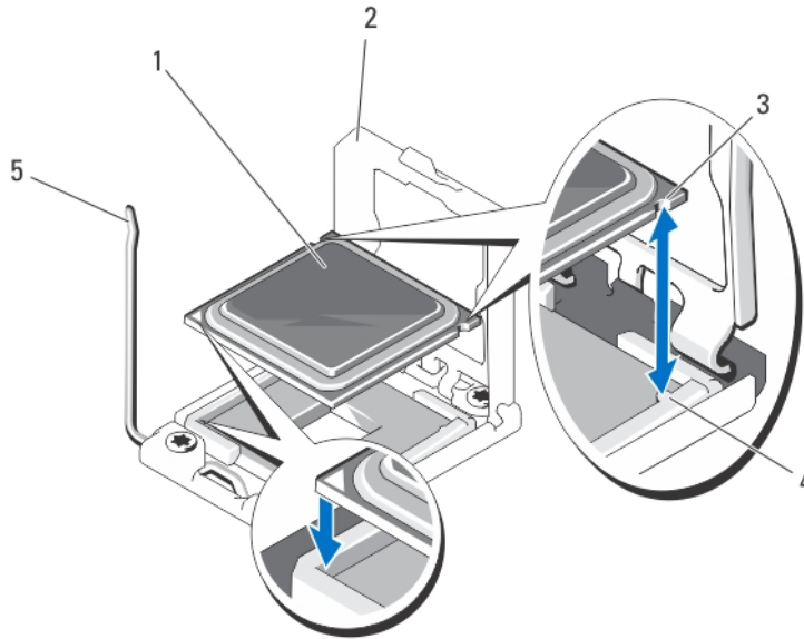
图 14: 卸下和安装处理器
