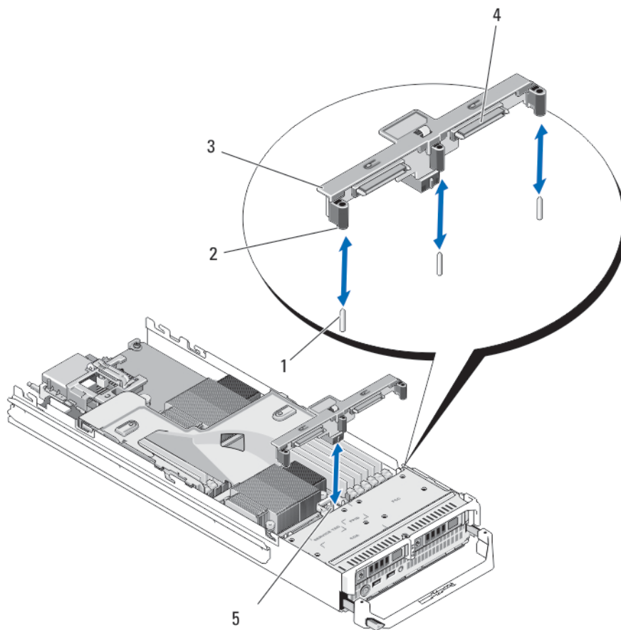
图 17: 卸下和安装硬盘驱动器/SSD 背板
