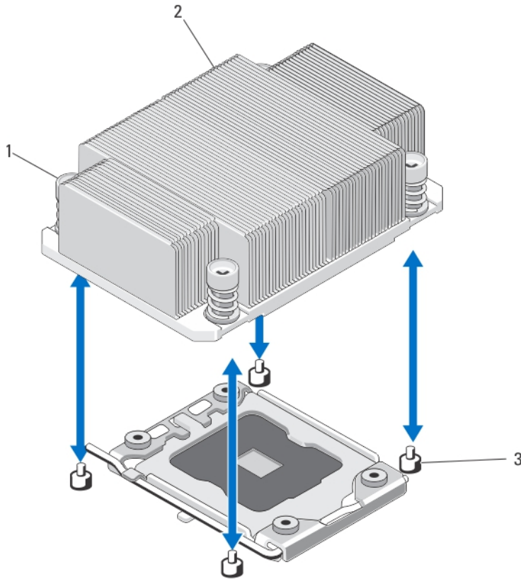
图 13: 卸下和安装散热器
