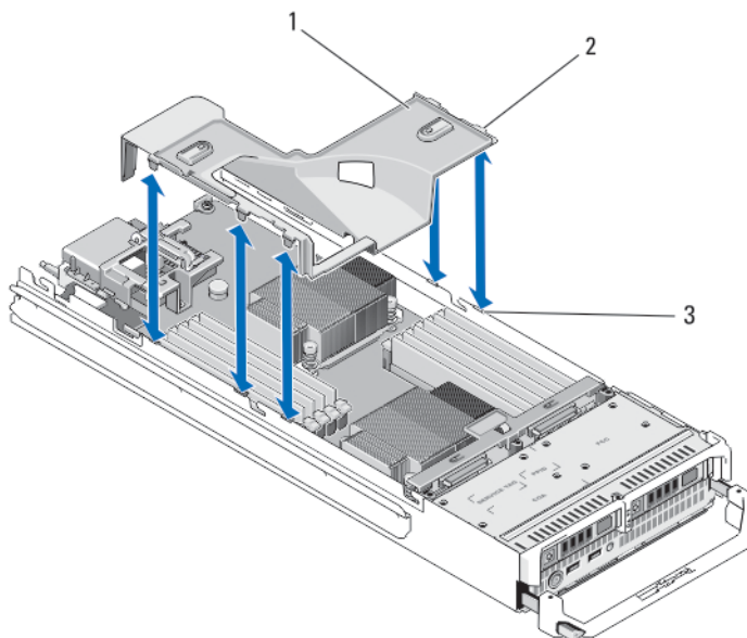
图 6: 卸下和安装冷却导流罩
