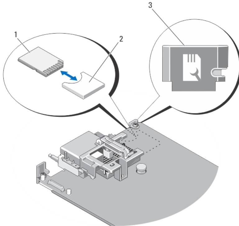
图 12: 装回 SD vFlash 卡
