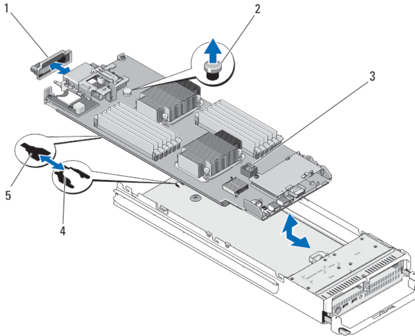
图 18: 卸下和安装系统板
