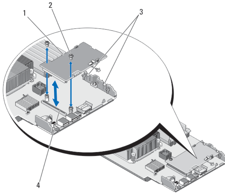
图 20: 卸下和安装存储控制器卡
