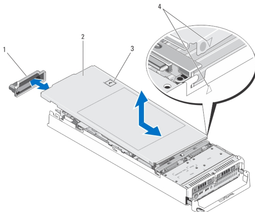
图 4: 打开与合上刀片
