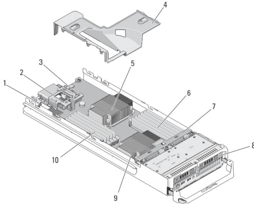
图 5: 刀片内部
