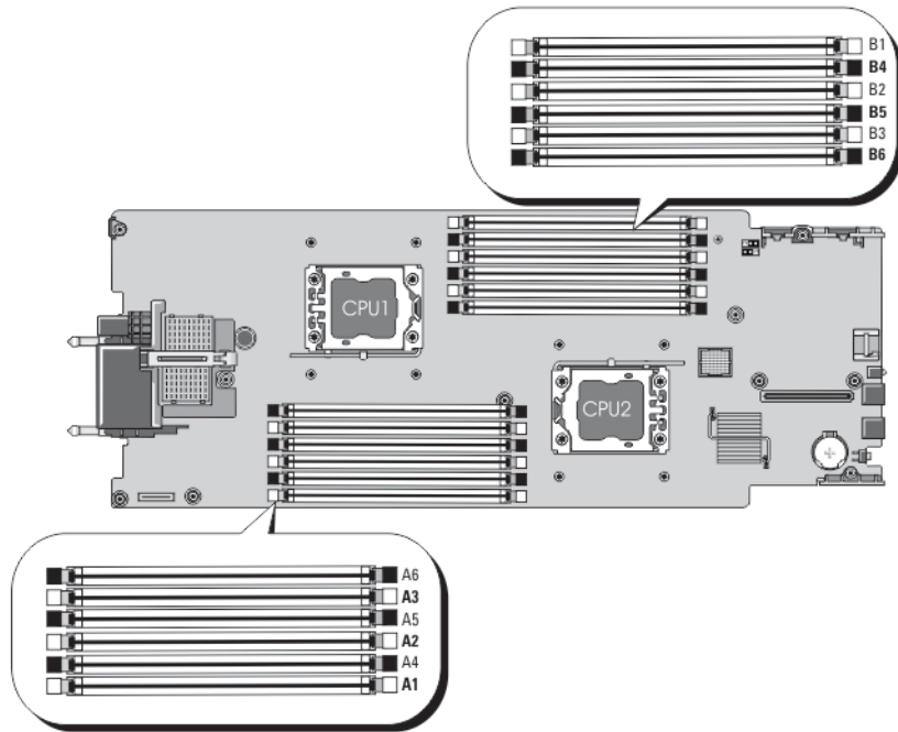
图 7: 内存插槽位置
