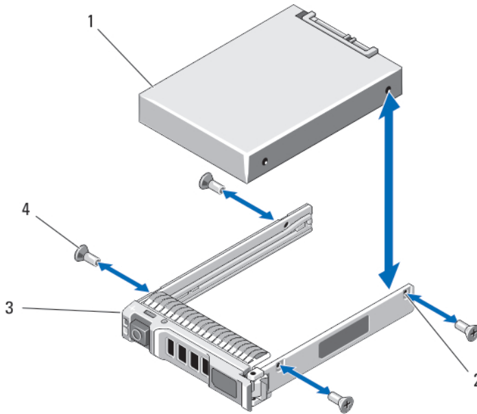
图 16: 在硬盘驱动器/SSD 托盘中卸下和安装硬盘驱动器/SSD
