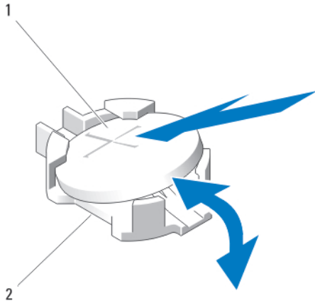
图 19: 更换 NVRAM 备用电池
